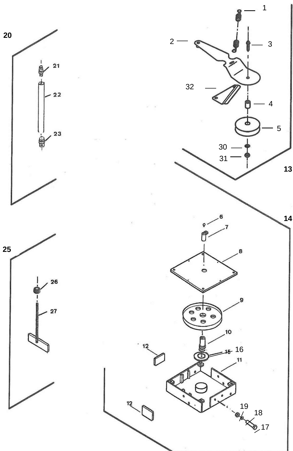
Figure 3. Hjørnerulle og Strammearm / Corner Roller and Tension Arm / Eckrolle und Spannenarm
