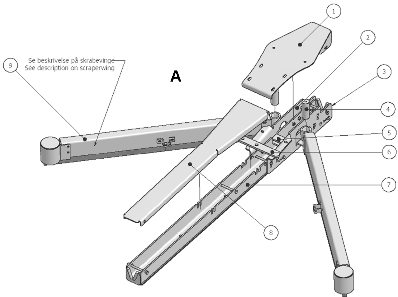
Figure 8. D70 Deltaskraber med plast / Delta scraper with plastic / Deltaschieber mit Kunststoffkufen
